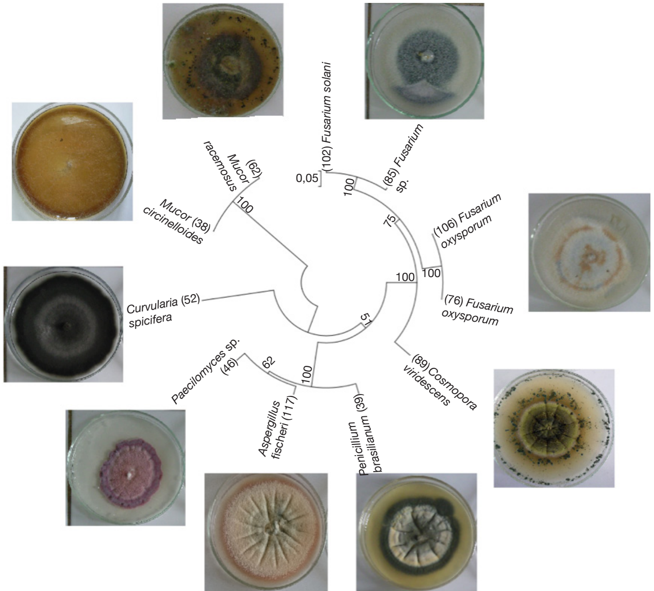
Figure 3. Phylogeny construction of the best performing ligno-cellulolytic species based on ITS sequences — Arbre phylogénétique des espèces ligno-cellulolytiques performantes basé sur les séquences ITS.
